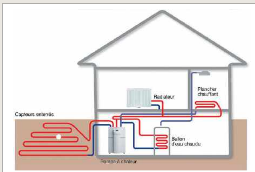
Schéma de fonctionnement d'une pompe à chaleur géothermique avec captage horizontal. Le captage horizontal est moins performant mais moins cher que le captage vertical (avec sondes).
